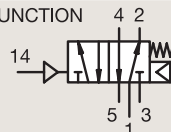
5/2 FUNCTION
