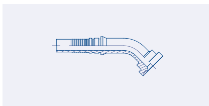
Interlock 45° Swept SAE 6000 PSI (code 62) Flange (SFS 45°) 26.7046 pag. 102
