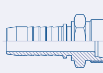
Male Metric Heavy Serie 24° Cone Seat (CES)
