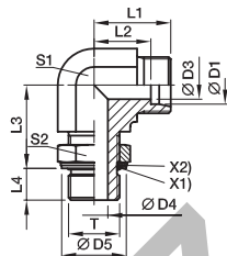
X1) O-kroužek OR X2) opěrný kroužek
